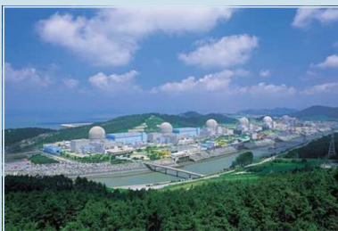
La centrale nucléaire de Yonggwang récemment renommée Hanbit, province de Jeolla du Sud, République de Corée. Crédit photo : Korea Hydro and Nuclear Power (KHNP)
